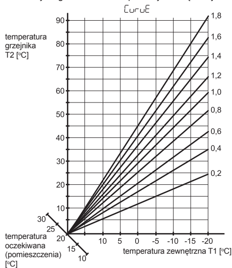
Krzywe grzewcze dla temperatury wewnętrznej 20 °C
